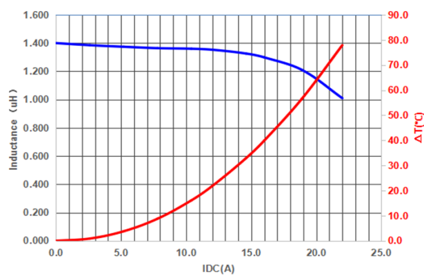
PIF0603A1R2MN
