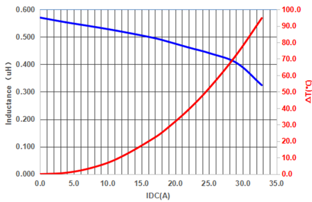
PIF0603AR56MN
