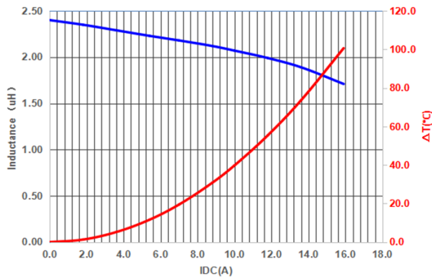
PIF0603A2R2MN
