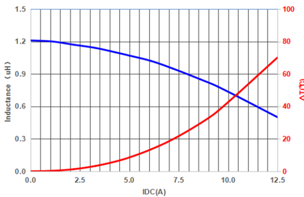
PIF0402LR1R2MN
