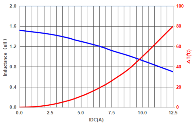
PIF0402LR1R5MN
