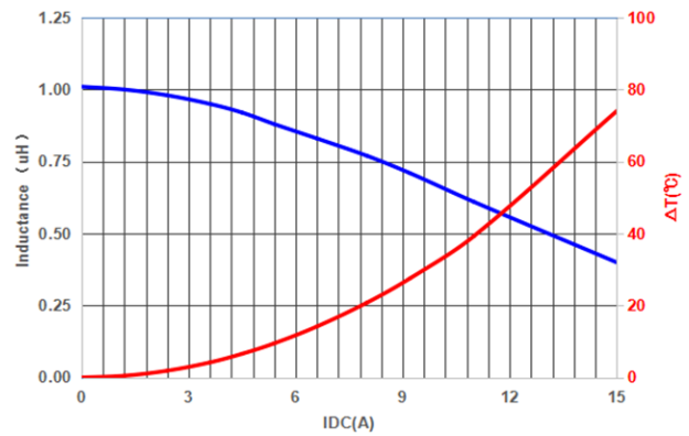
PIF0402LR1R0MN
